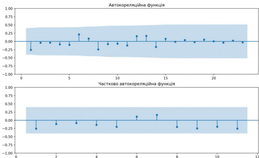
Рис. 2 Графіки АКФ та ЧАКФ
