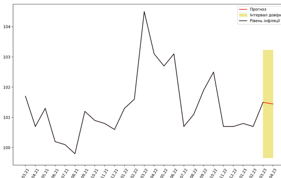
Рис. 3 Прогноз рівня інфляції на квітень 2023 р
